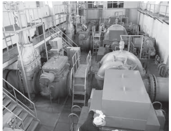
フル稼働した笹川揚水機場のポンプ。3台のポンプは来年2月末までに新しいポンプと入れ替わる予定
